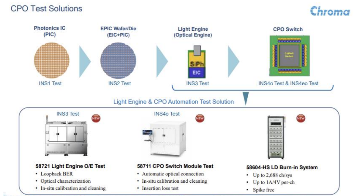
圖 3：致茂 2H26 預計出貨之 Insertion 4 CPO Tester (圖中間)
